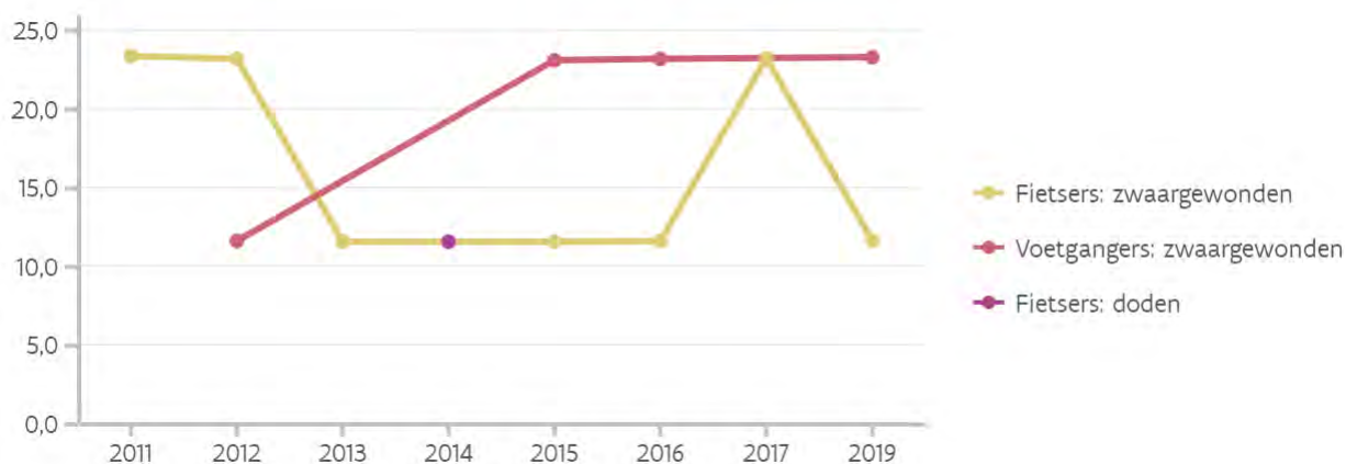
Verkeersslachtoffers bij fietsers en voetgangers, 2011-2020, in aantal slachtoffers per 100.000 inwoners (Merksplas)
